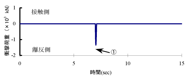
図-23 桁間の衝撃力の時刻歴応答(Case6)
