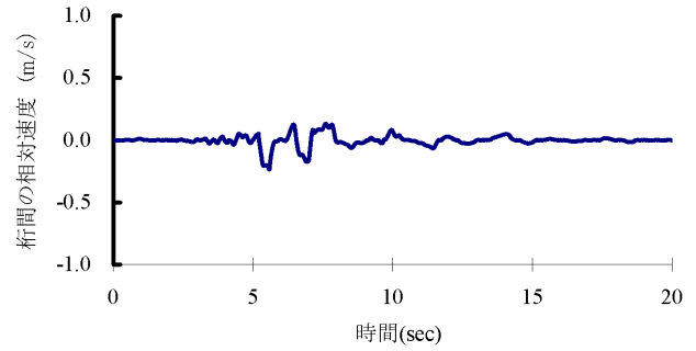
図-24 Case7の時刻歴応答図
