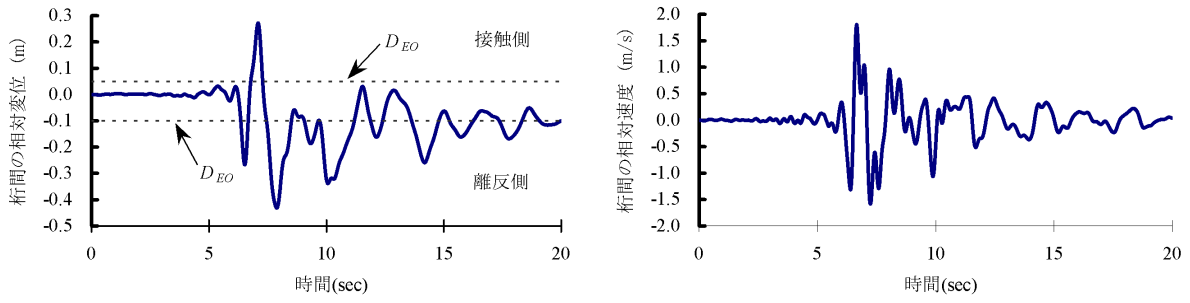
図-12 Case1の時刻歴応答図
