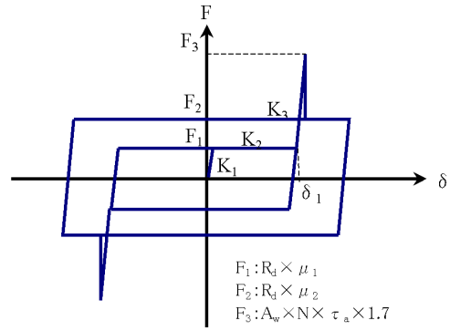
図-8 可動支承の復元力モデル
