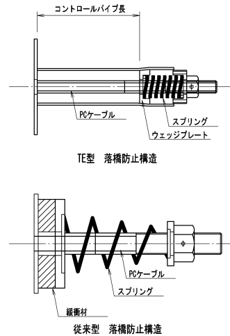
図-2 TE型と従来型の構造
