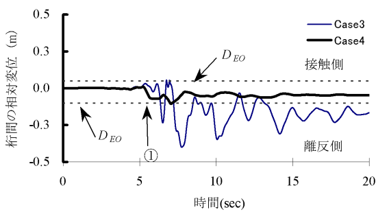
図-20 相対変位の時刻歴応答図
