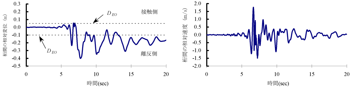
図-13 Case3の時刻歴応答図
