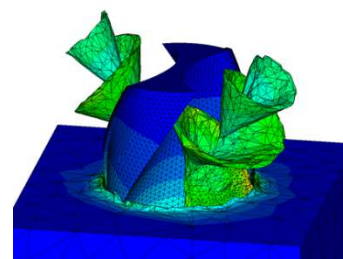
AdvantEdge によるドリル加工解析
