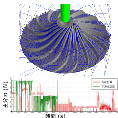
Production Module による インペラ加工解析
